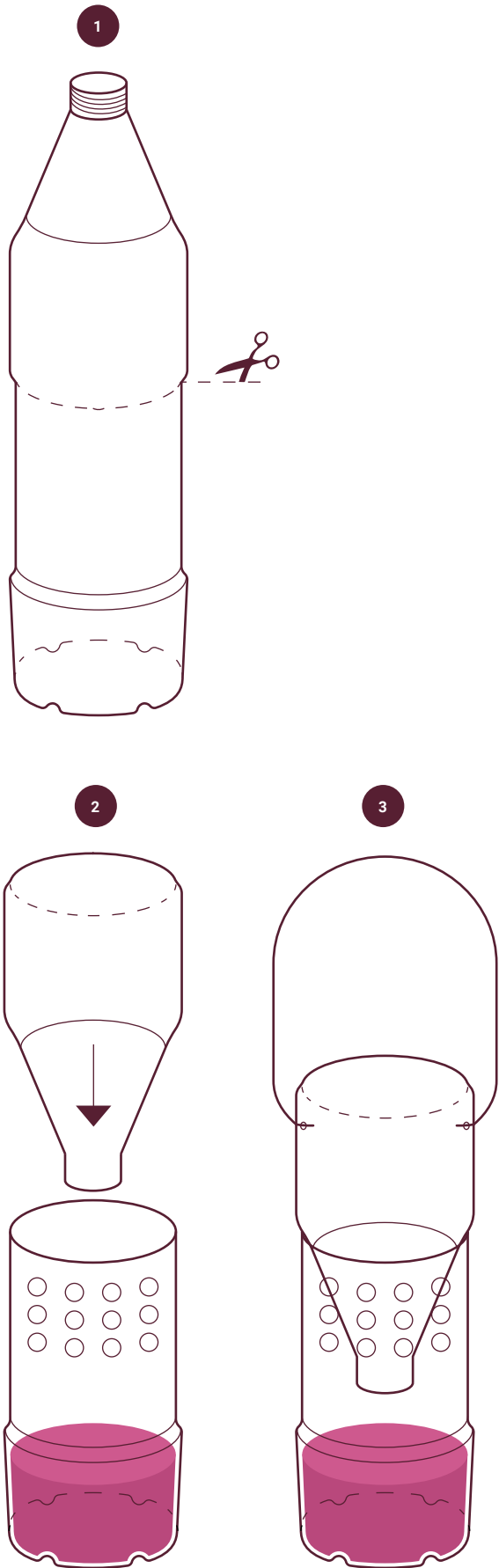
Obr. 3: Postup výroby pastí na odchyt sršní [upraveno dle Mairie Châteaubriant 2021].
